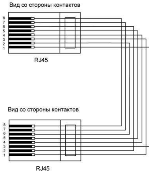
Рисунок Б.1 – Схема кабеля Ethernet Crossover
